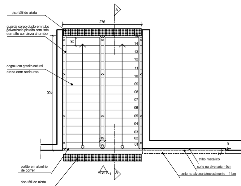
PLANTA ESCADA DE ACESSO
