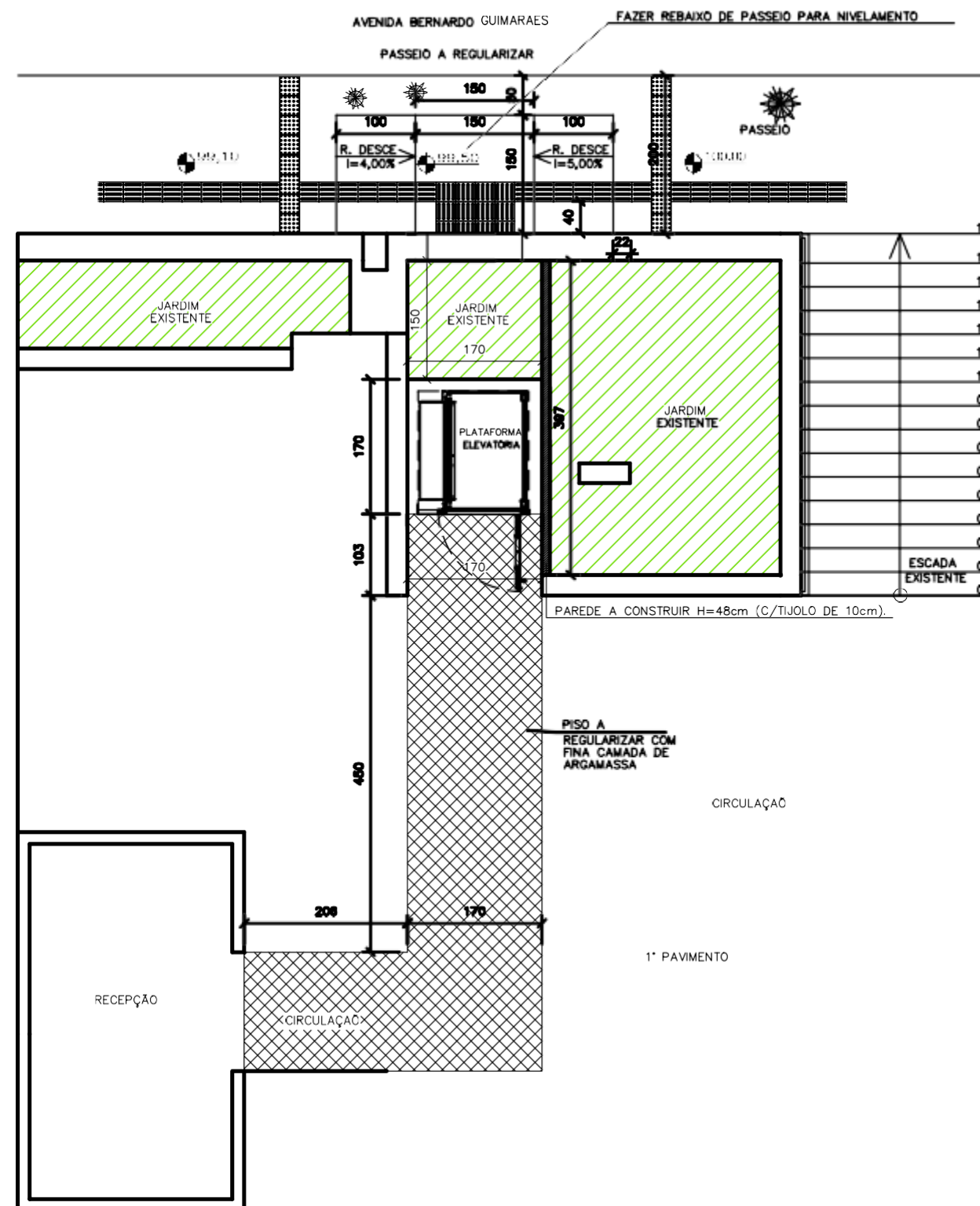
PLANTA DO 1º PAVIMENTO – A CONSTRUIR ESC: 1:75
