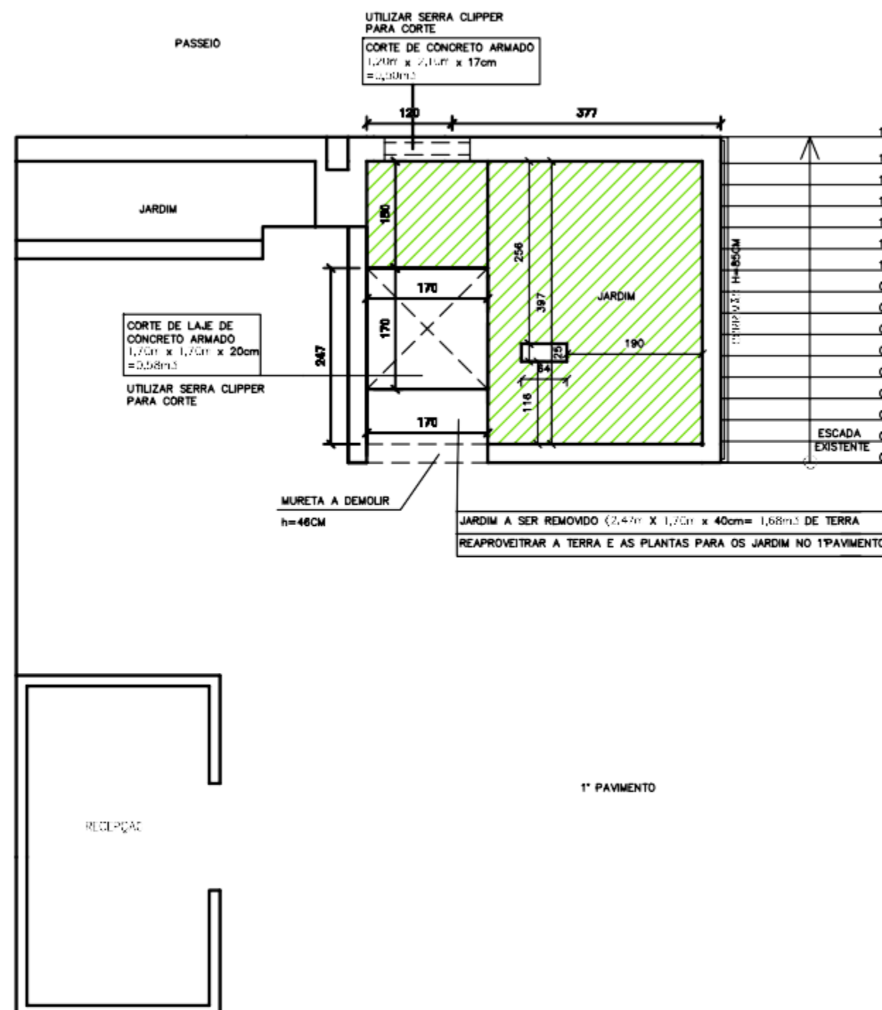
PLANTA DO 1º PAVIMENTO – DEMOLIÇÃO ESQ: 1275
