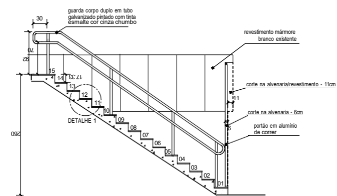
CORTE A-A
