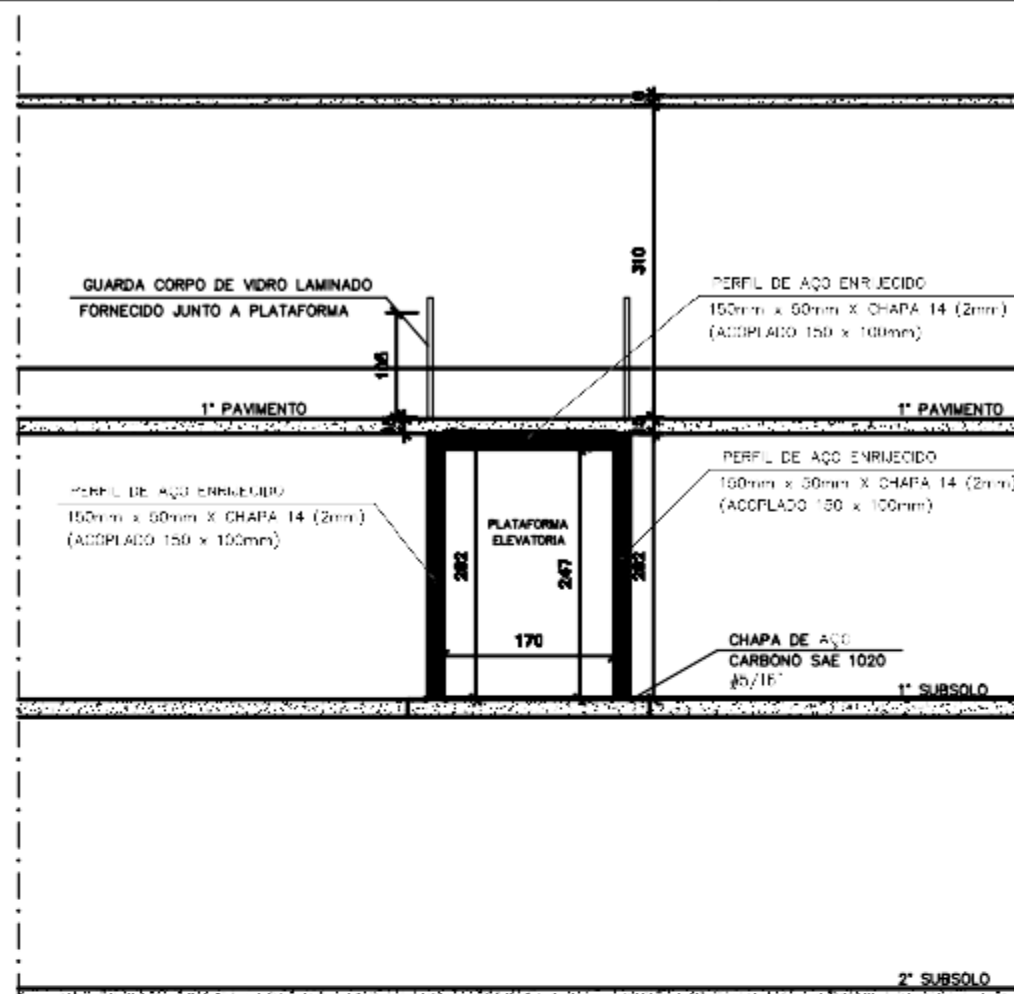
DETALHE REFORÇO ESTRUTURAL ESC: 1:75
