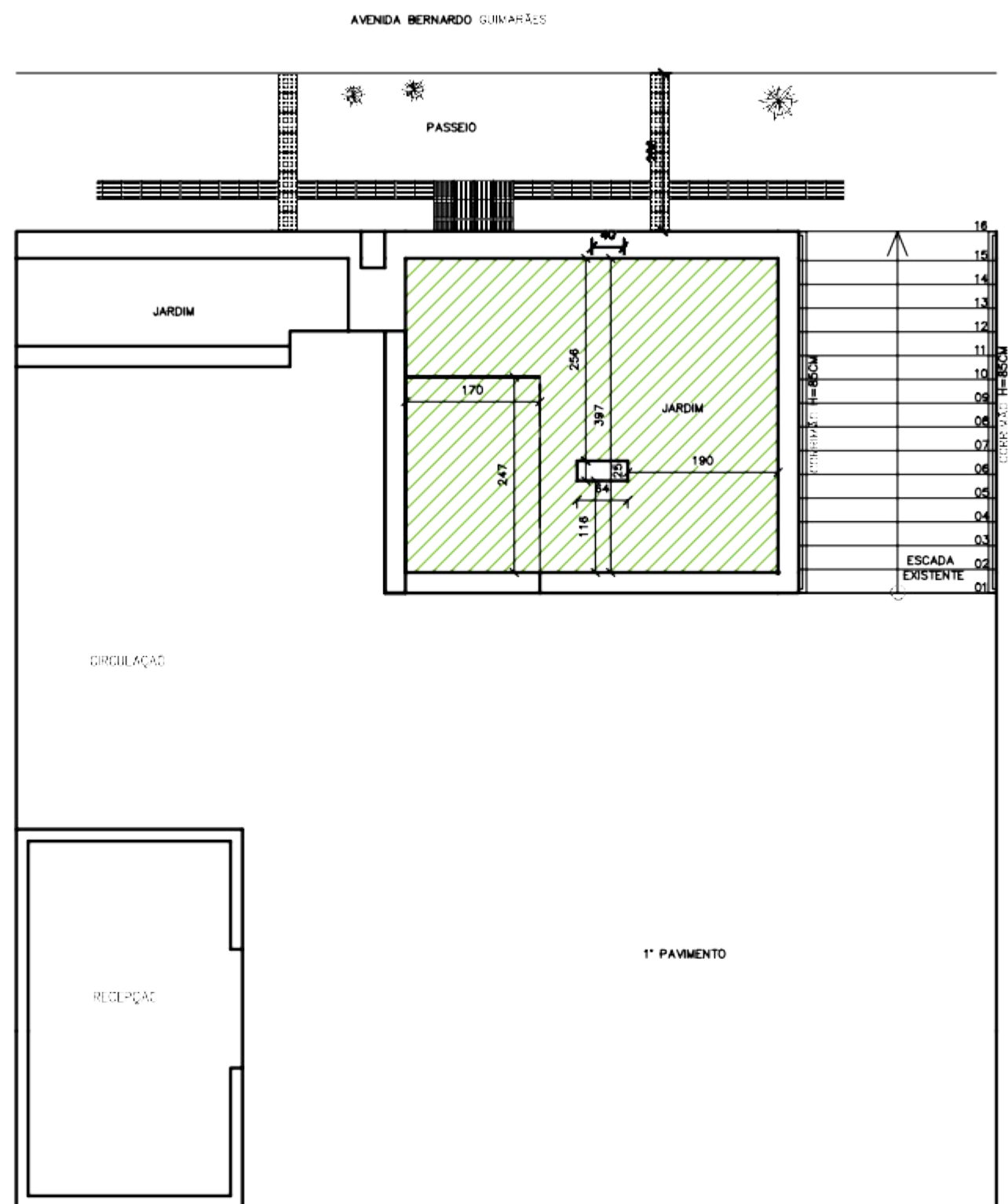
PLANTA DO 1º PAVIMENTO EXISTENTE ESC.: 1:75
