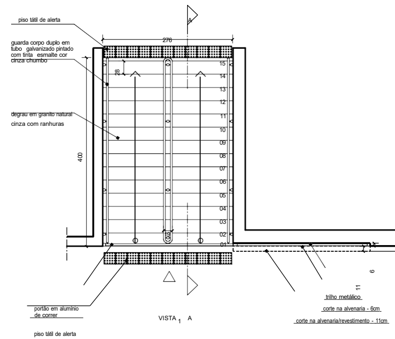
PLANTA ESCADA DE ACESSO
