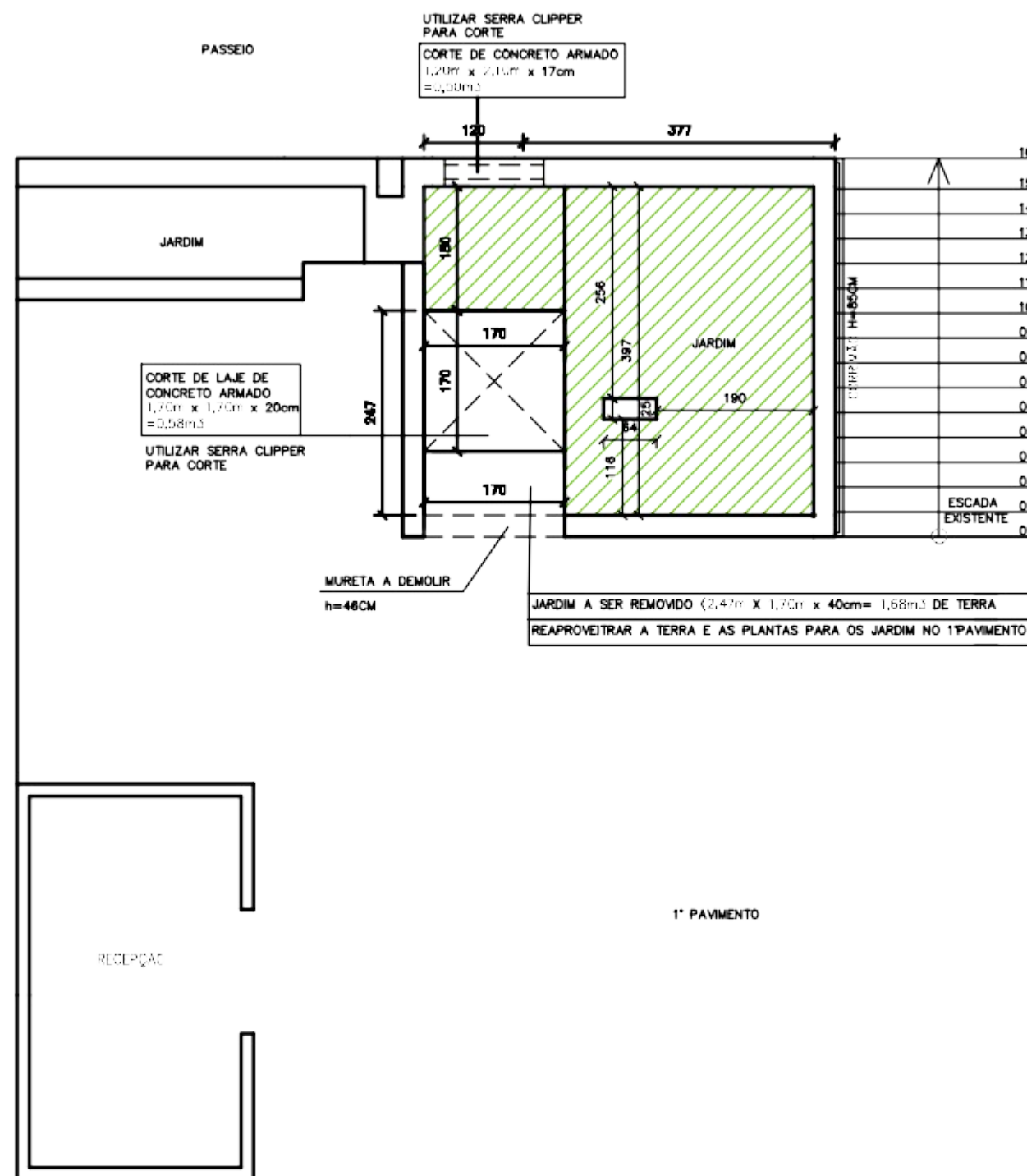
PLANTA DO 1º PAVIMENTO – DEMOLIÇÃO ESC.: 1:75
