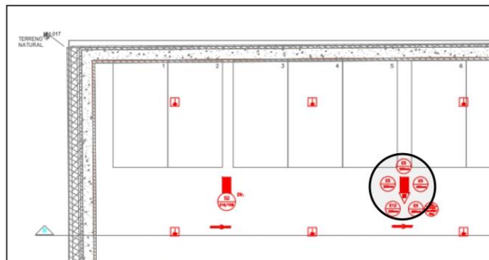
Figura 4 – Extintor a ser instalado no 1º subsolo
