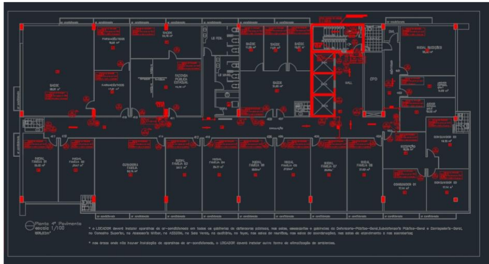
Imagem 5 - Layout antigo; 4º Pavimento
