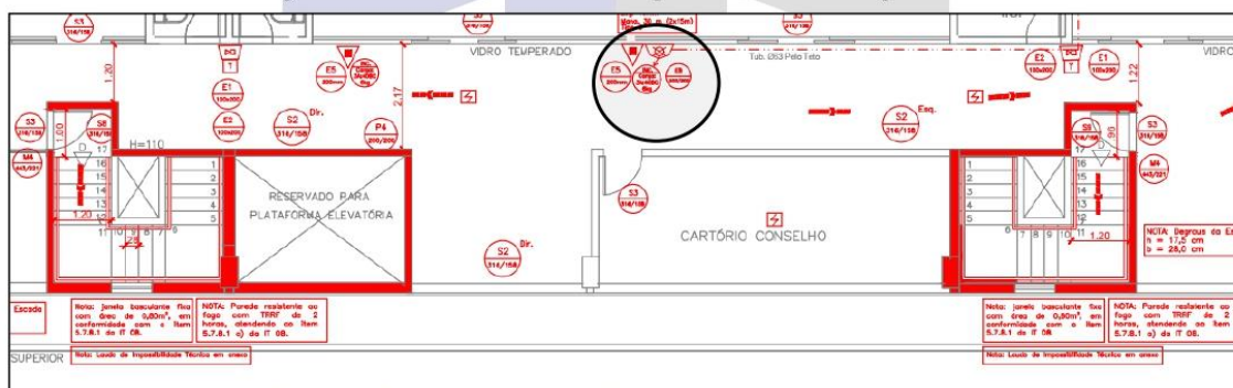
Figura 7 - Escadas enclausuradas e novo ponto de hidrante no 8º pavimento
