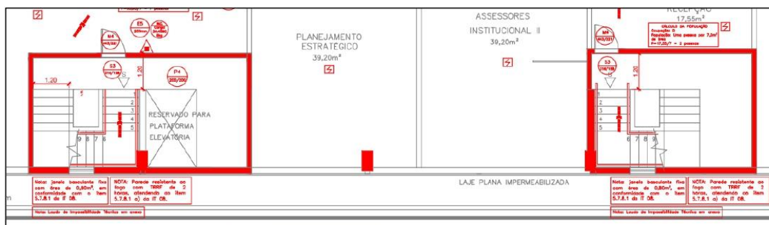
Figura 6 - Escadas enclausuradas no 7º pavimento
