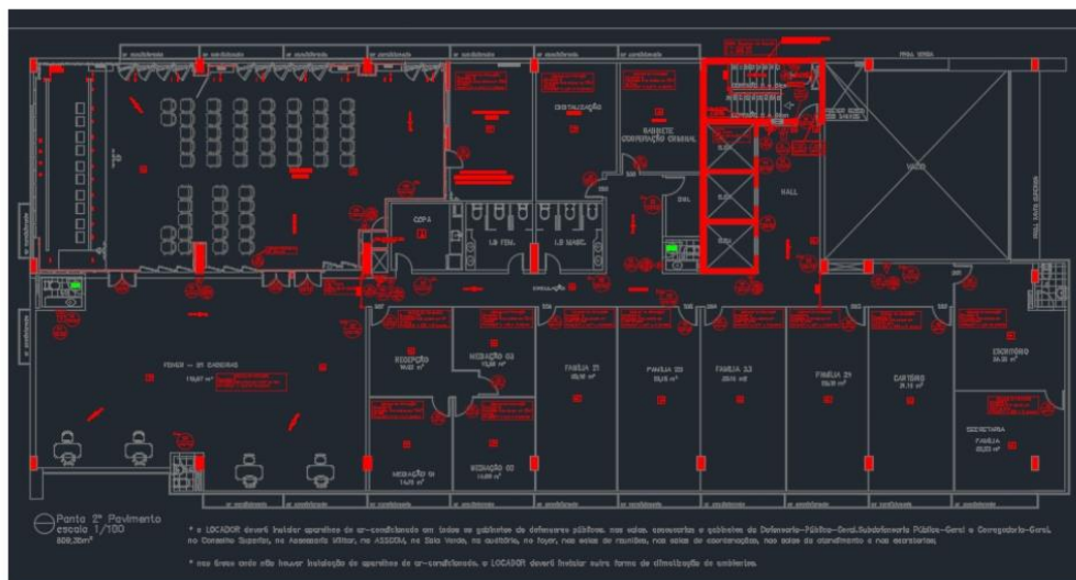
Imagem 3 - Layout antigo; 2º Pavimento
