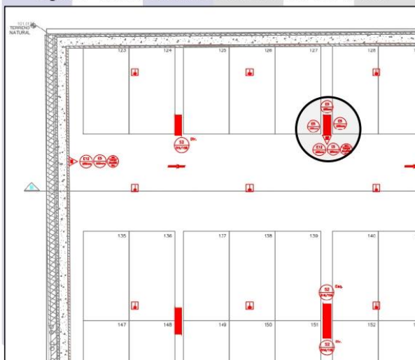
Figura 3 - Extintores a serem instalados no 3º e 2º subsolo
